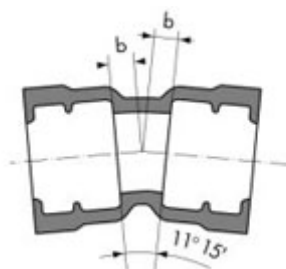
CURVA A DUE BICCHIERI 11° 15' (1/32)
