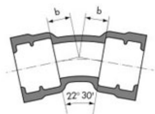
CURVA A DUE BICCHIERI 22° 30' (1/16)
